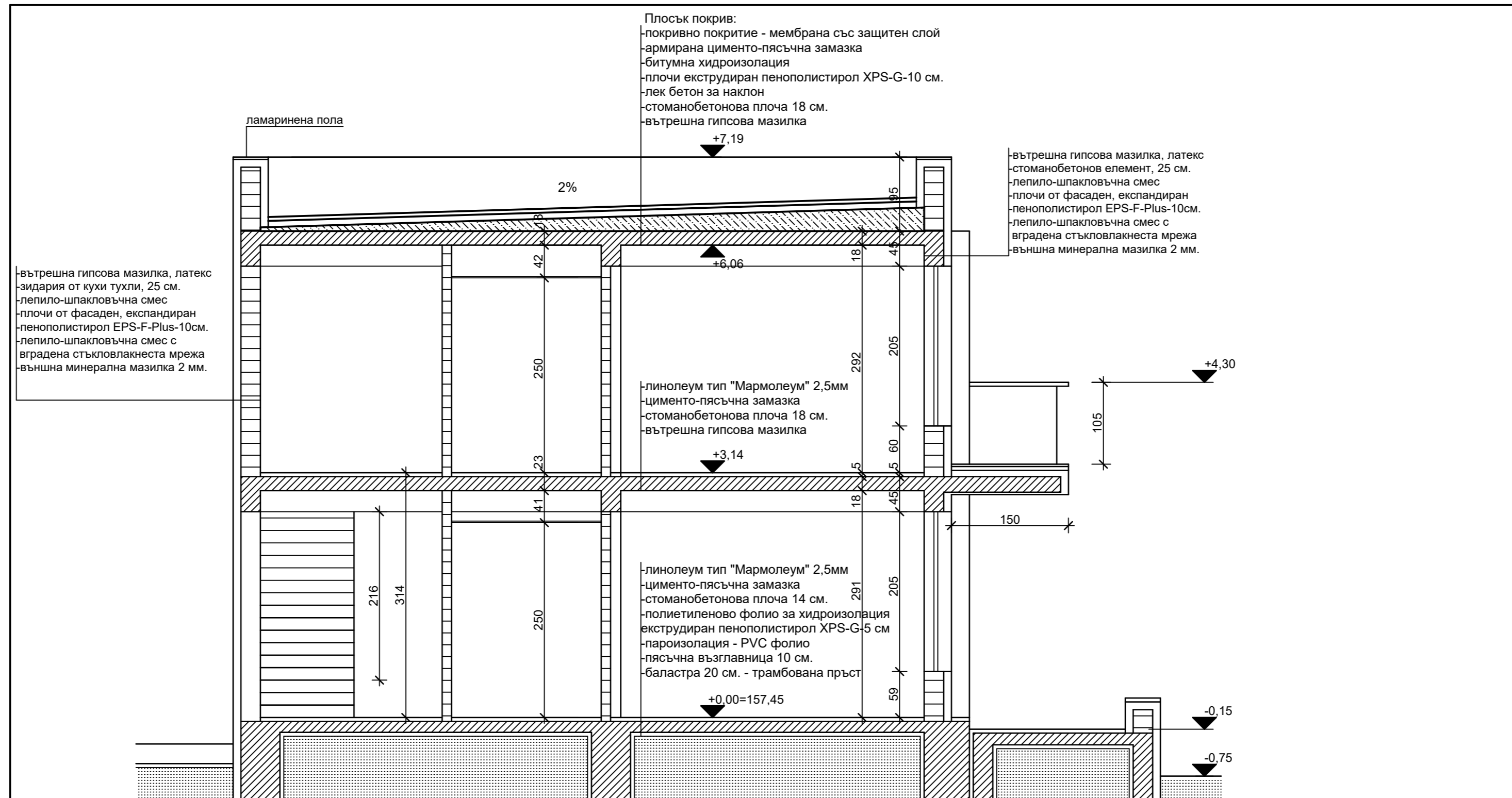
РАЗРЕЗ 1-1 М 1:50
